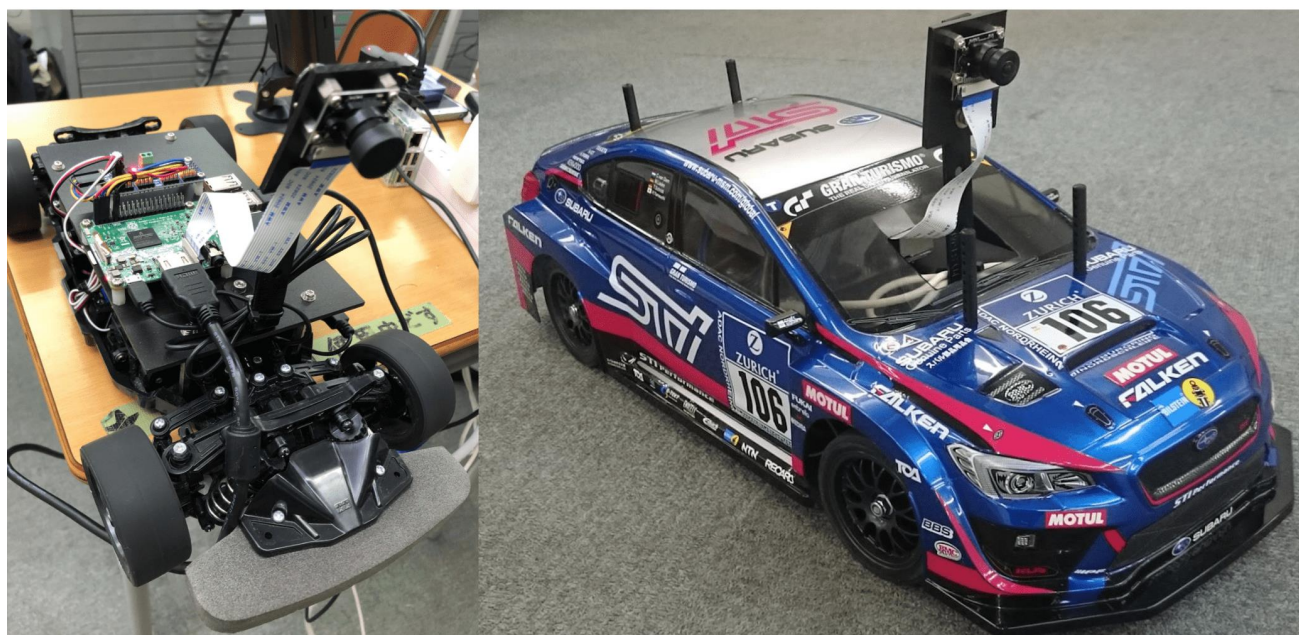
Raspberry Pi を搭載した TAMIYA 製ラジコンカー
